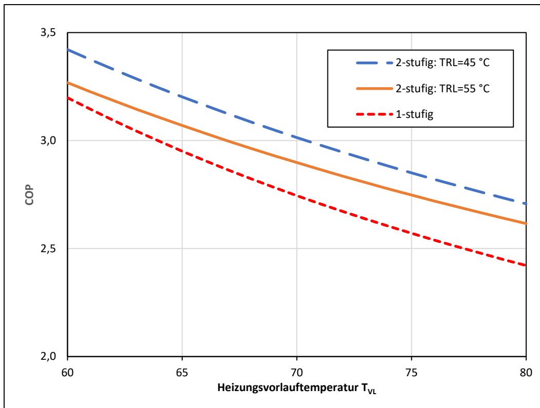
Abbildung 22: COP in Abhängigkeit der Heizungsvorlauftemperatur bei 1-stufiger und 2-stufiger Ausführung und einer Quelltemperatur von T_a = 10 °C.
