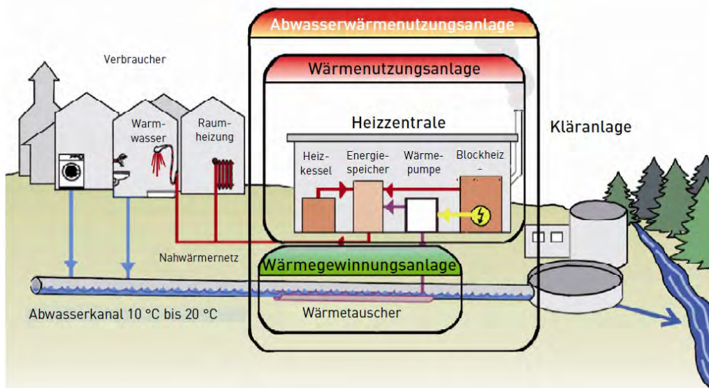
Abbildung 3: Aufbau einer Abwasserwärmenutzungsanlage (DWA-Merkblatt M114, 2020).
