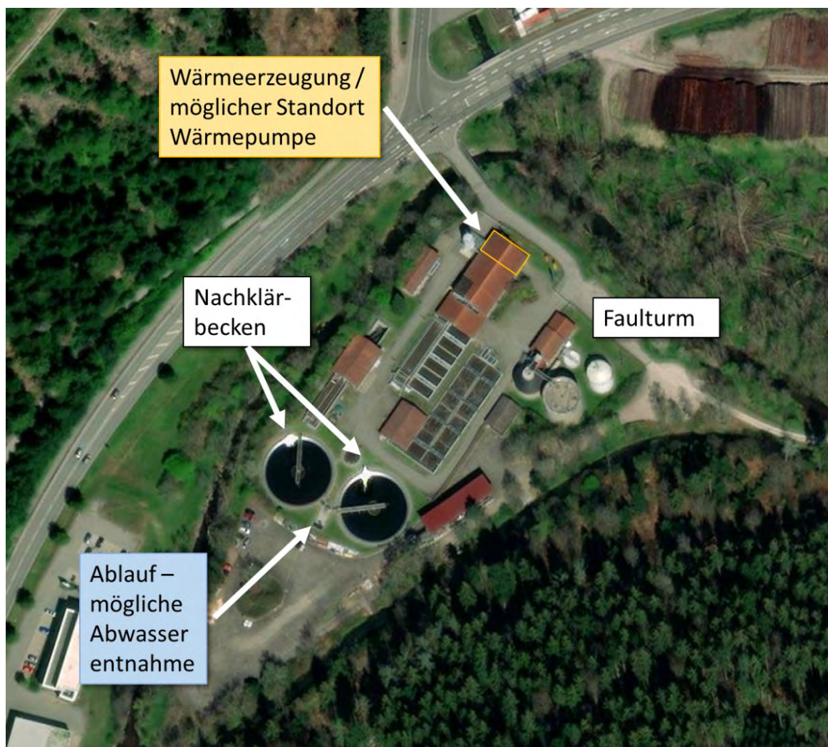
Abbildung 34: Luftbild und geplante Umsetzung des technischen Konzepts auf der Kläranlage Altensteig. Bildquelle: esri / ArcGIS.
