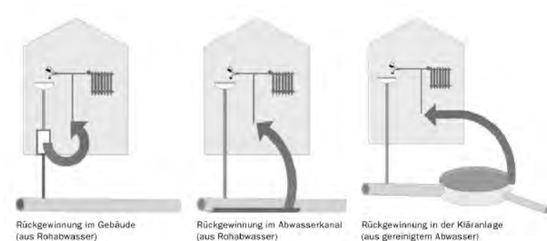
Abbildung 2: Mögliche Entnahmepunkte der Wärme aus dem Abwasser (Müller & Schmid, 2005).
