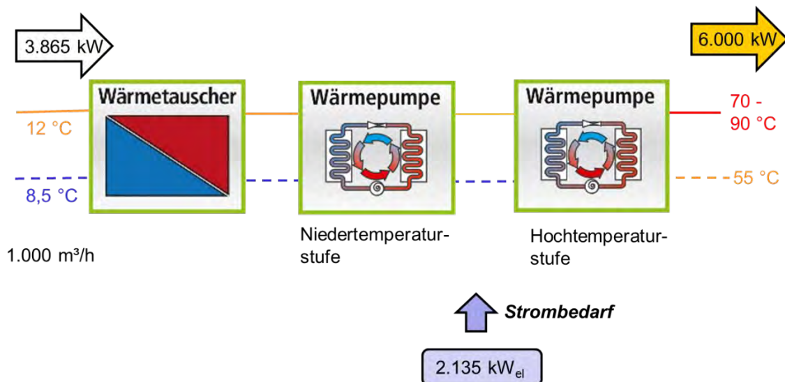
Abbildung 26: Konzept zur zweistufigen Wärmeauskopplung.
