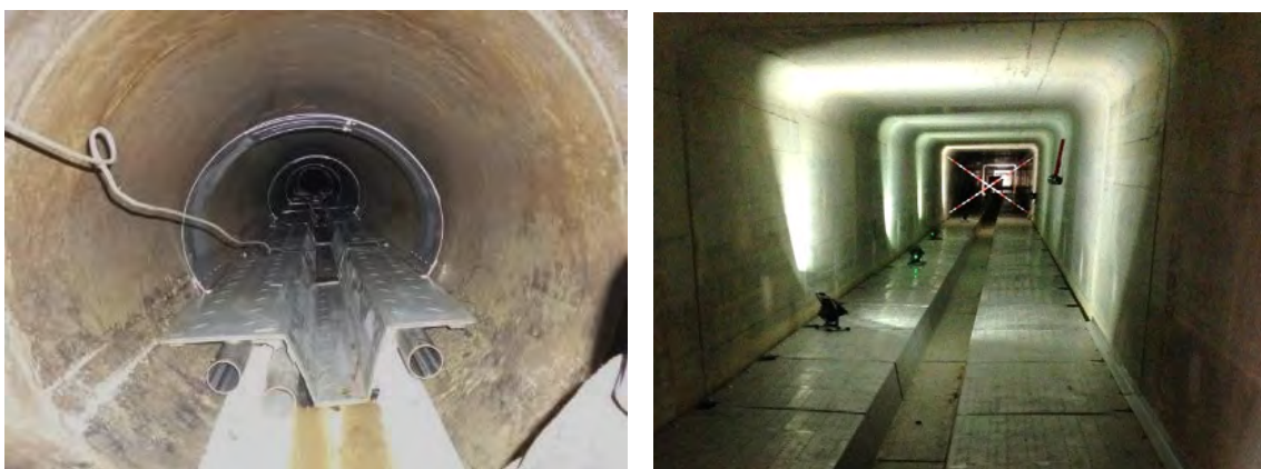
Abbildung 18: Foto links: Einbau Wärmetauscher in kleineren bestehenden Rundkanal. Foto rechts: Einbau Wärmetauscher in einen größeren Rechteckkanal im Zuge des Kanalneubaus. Quelle: IBS.
