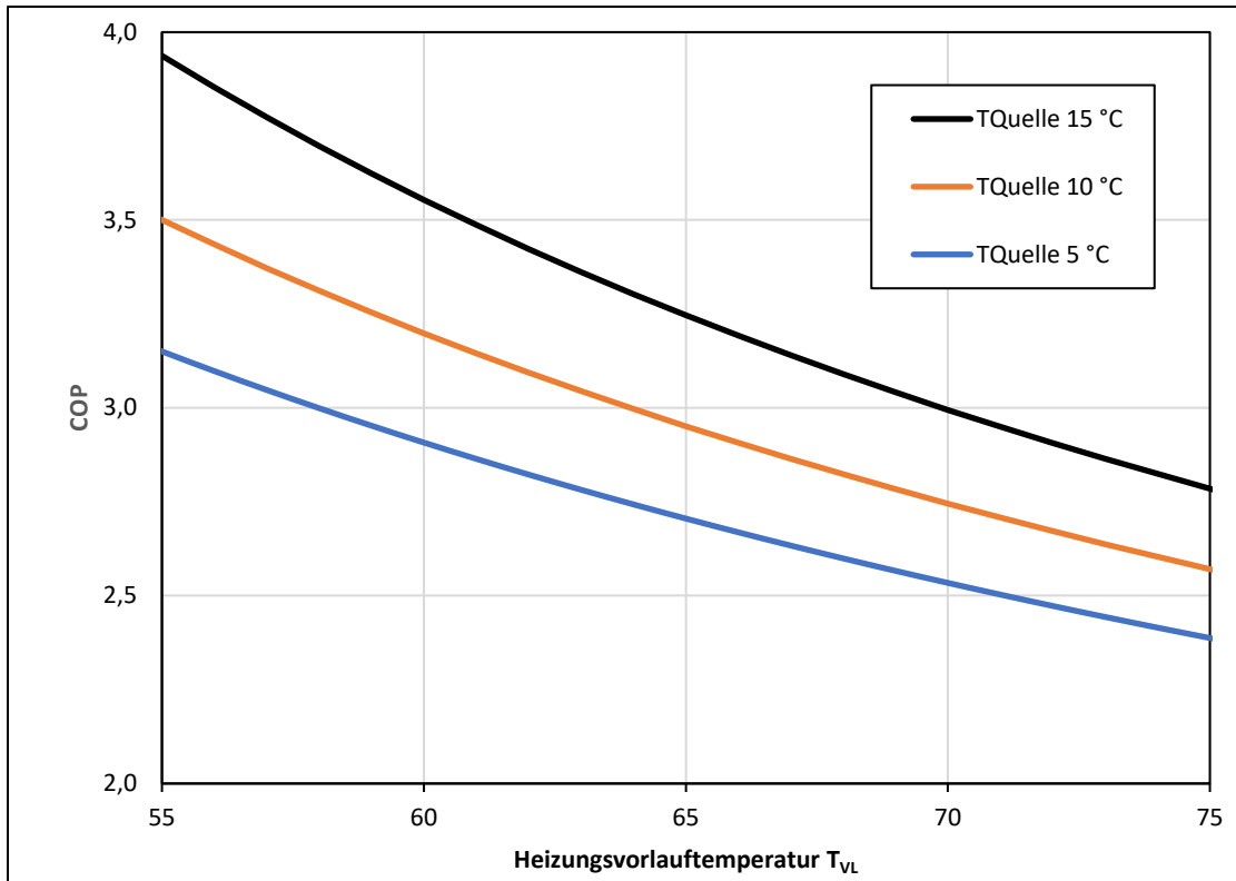
Abbildung 21: COP einer Wärmepumpe in Abhängigkeit der Heizungsvorlauf- und Wärmequelle-temperatur.
