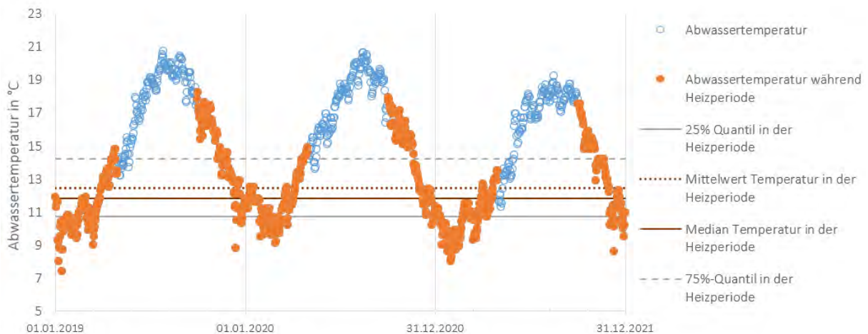
Abbildung 39: Ganglinie der Abwassertemperatur und Kenngrößen der Abwassertemperatur während der Heizperiode an einem Beispiel-Standort.
