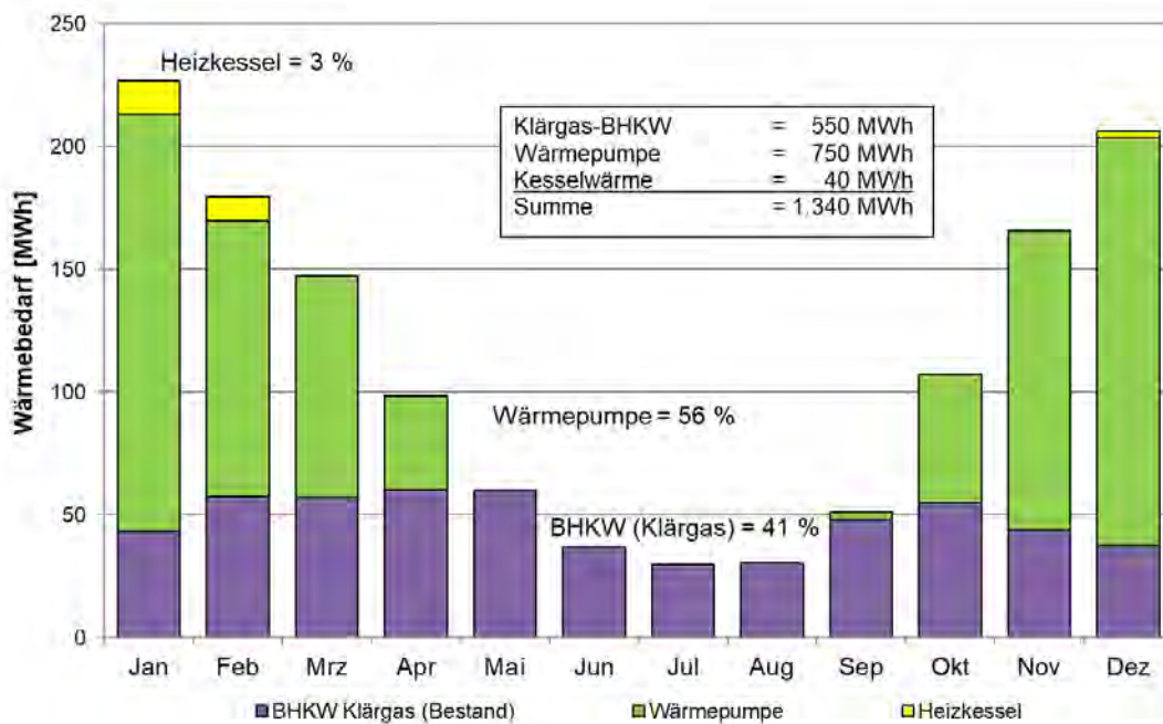
Abbildung 36: Monatsbilanz Deckung Wärmebedarf gemäß Konzept.
