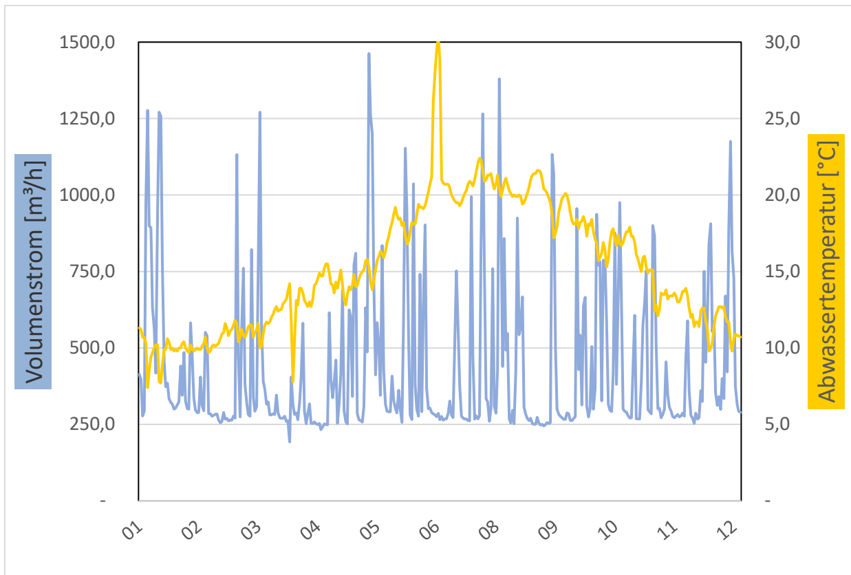
Abbildung 31: Verlauf Abwasservolumenstrom und -temperatur über das Jahr am Standort Weinstadt.
