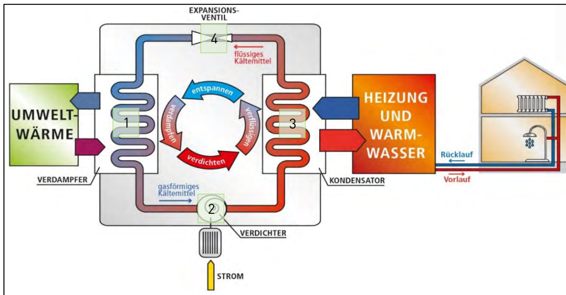
Abbildung 15: Der Wärmepumpen-Kreislaufprozess. Quelle: IBS.
