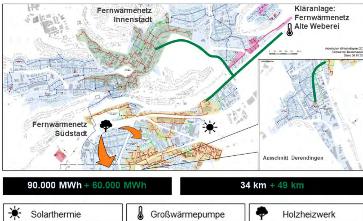
Abbildung 29: Geplanter Netzverbund Süd. Bildquelle: Stadtwerke Tübingen.
