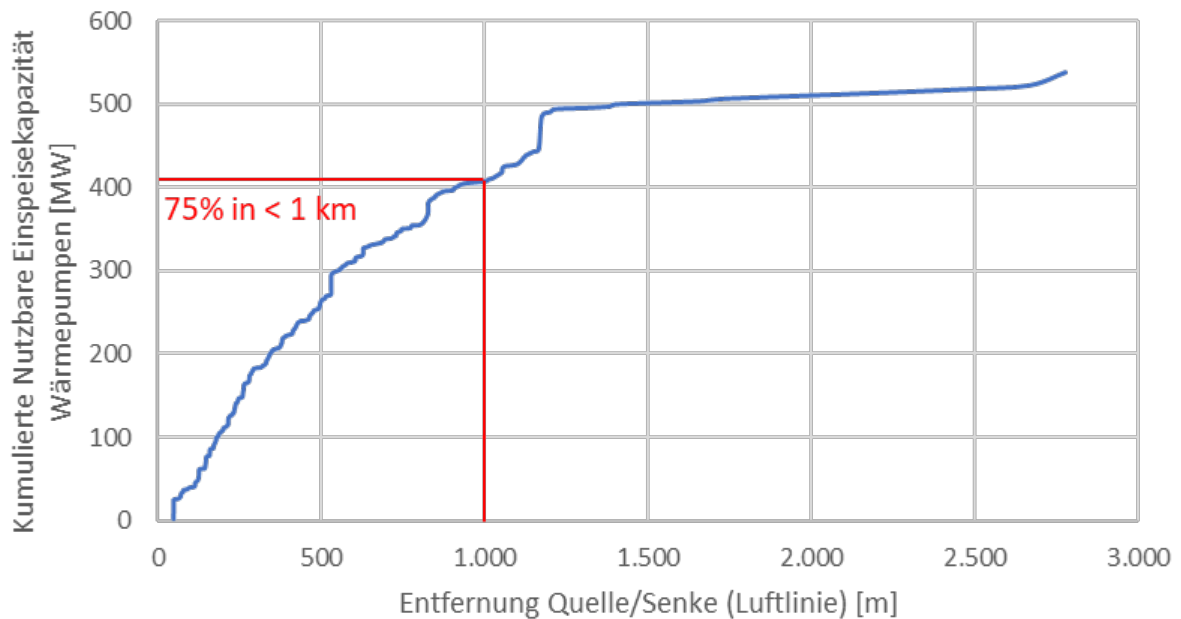
Abbildung 13: Entfernungspotenzialkurve.
