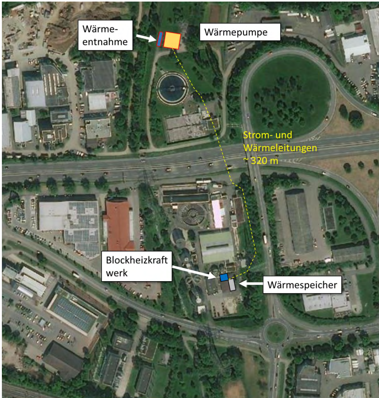
Abbildung 32: Konzept zur Nutzung der Abwasserwärme in Weinstadt. Bildquelle: esri / ArcGIS.
