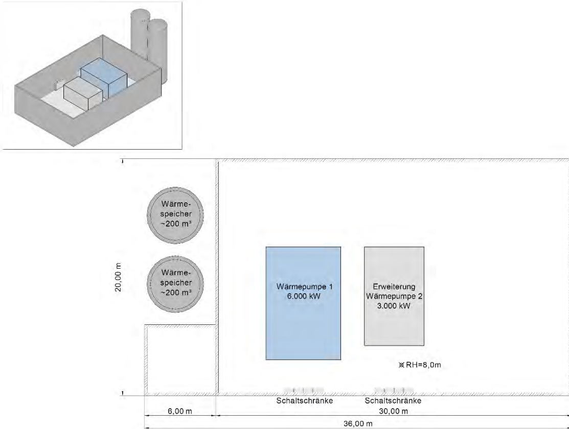
Abbildung 28: Aufstellungsplan und Platzbedarf.
