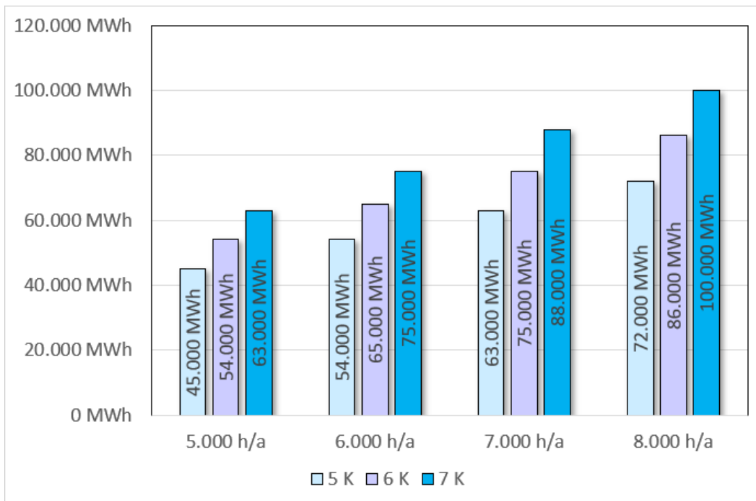
Abbildung 25: Potenzial zur Wärmeerzeugung bei verschiedenen Abkühlungen.
