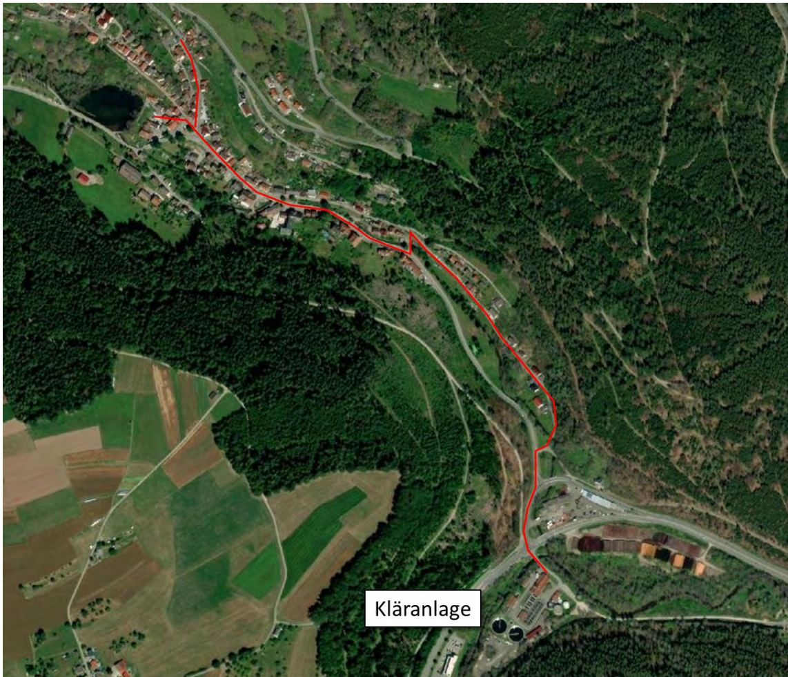
Abbildung 35: Übersicht des möglichen Wärmenetzes zur Versorgung des Teilorts Altensteig-Berneck. Bildquelle: esri / ArcGIS.
