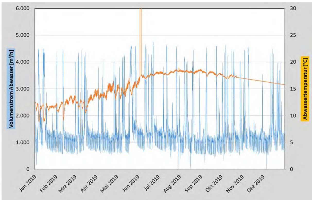
Abbildung 24: Verlauf Abwasservolumenstrom und -temperatur über das Jahr am Standort Tübingen.
