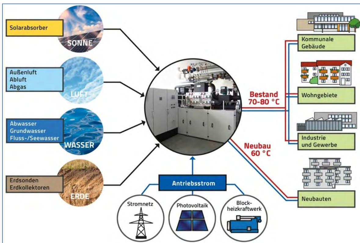
Abbildung 16: Wärmequellen, Antriebsenergien und Wärmeverbraucher. Quelle: IBS.
