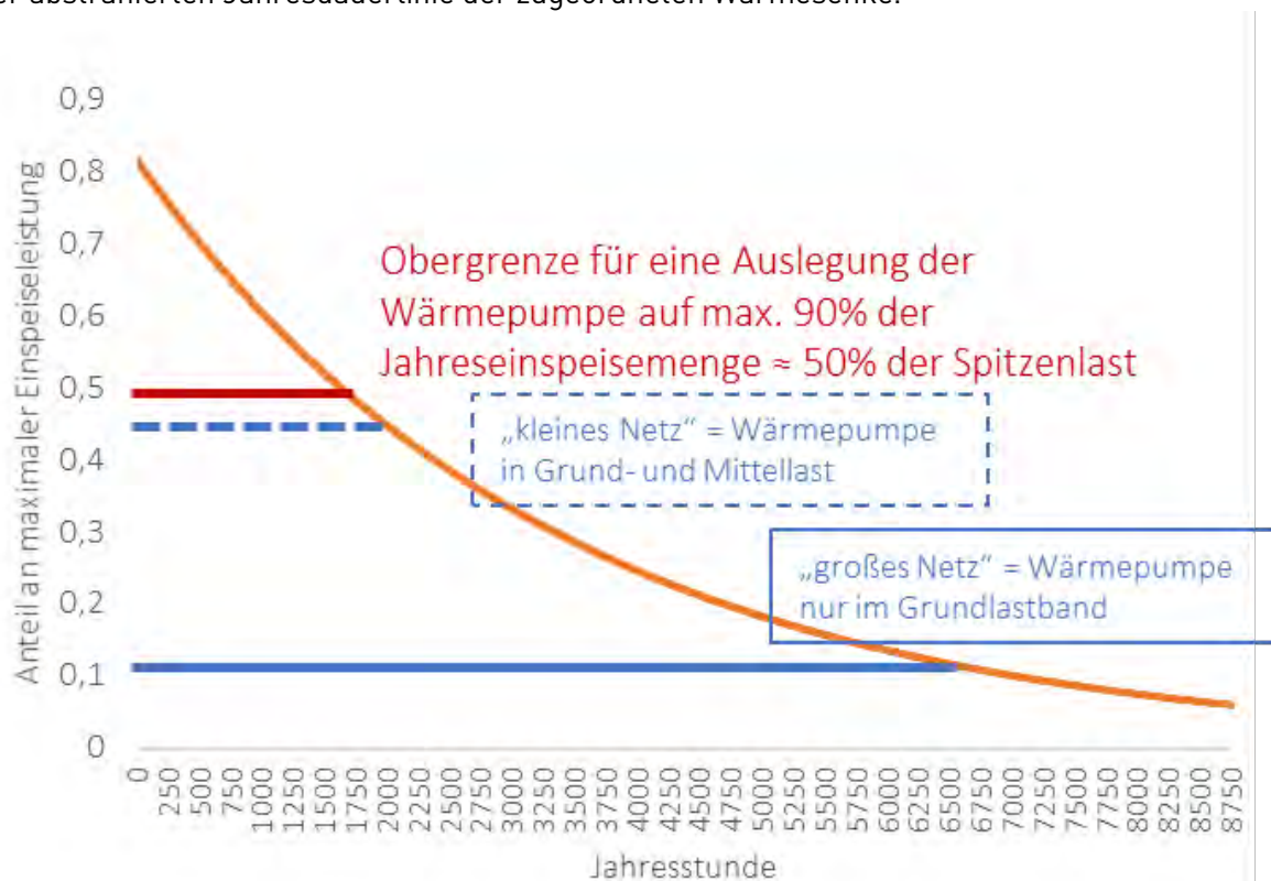
Abbildung 9: Nutzbare Einspeiseleistung und Wärmemenge im Abgleich mit der Jahresdauerlinie der zugeordneten Wärmesenke. Quelle: ifeu.
