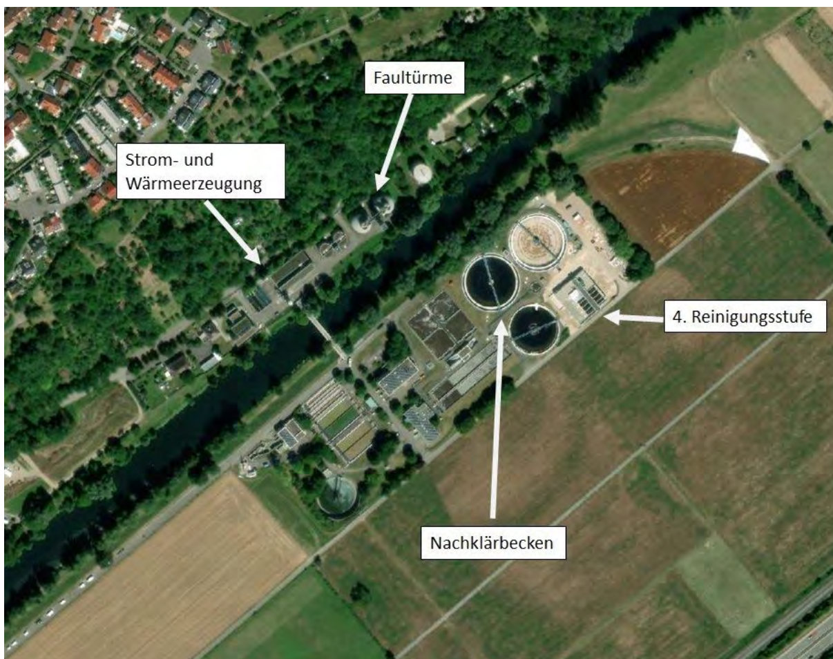
Abbildung 23: Luftbild Kläranlage Tübingen. Bildquelle: esri / ArcGIS.
