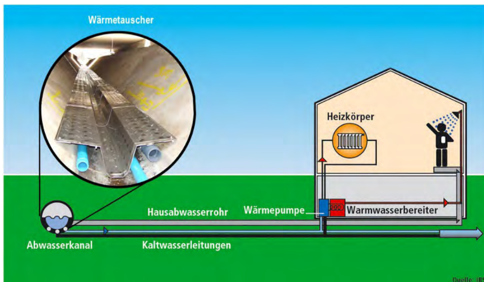
Abbildung 17: Prinzip der Abwasserwärmenutzung mit Wärmetauscher im Abwasserkanal. Quelle: IBS.
