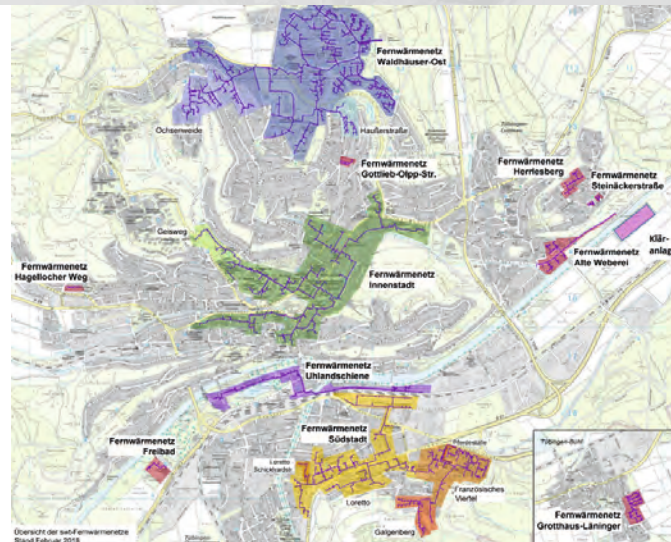
ABBILDUNG 1: ÜBERSICHT DES WÄRMENETZES TÜBINGEN
