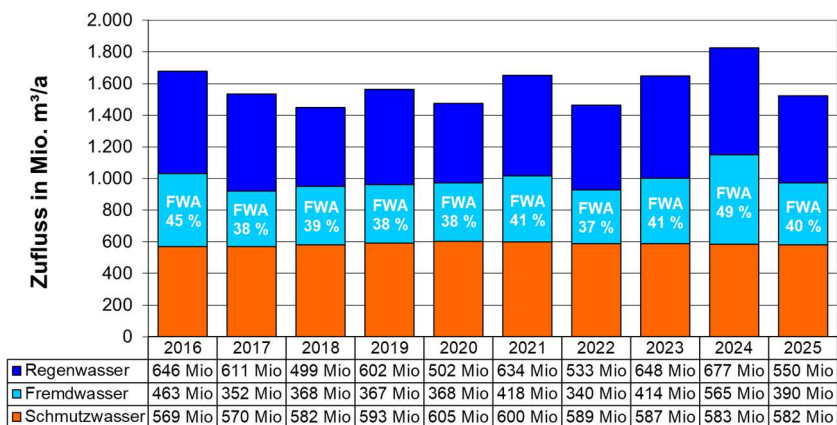
Abbildung 4: Zeitliche Entwicklung der behandelten Abwassermenge (Schmutz-, Fremd- und Regenwasserabfluss) (n = 841)
